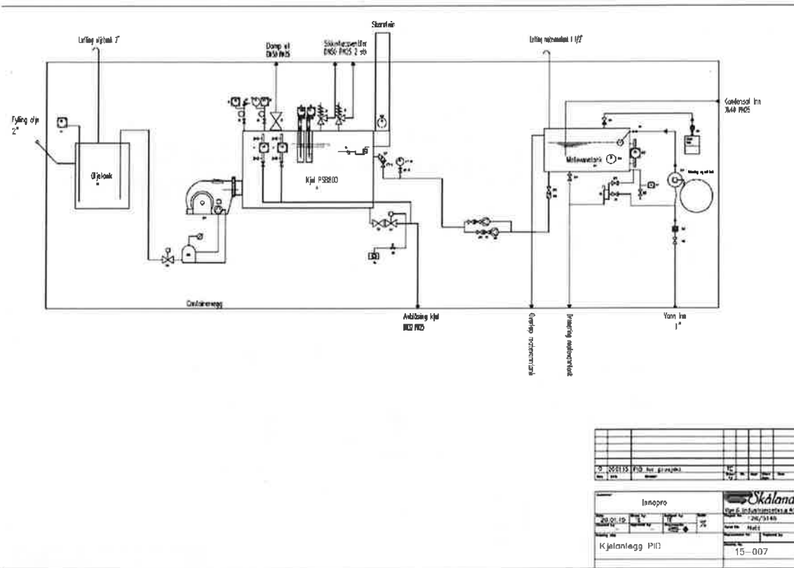
Bilde: 2: Dampkjele system
